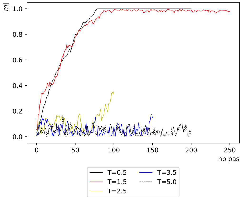
Evolution de l'aimantation sur critère Estimation par intervalle, N=32
